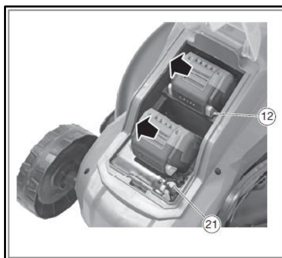
Obrázok 6: Priestor pre akumulátory vrátane akumulátorov
