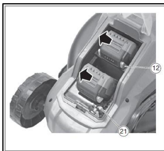
Obrázek 6: Přihrádka na akumulátory včetně akumulátorů
