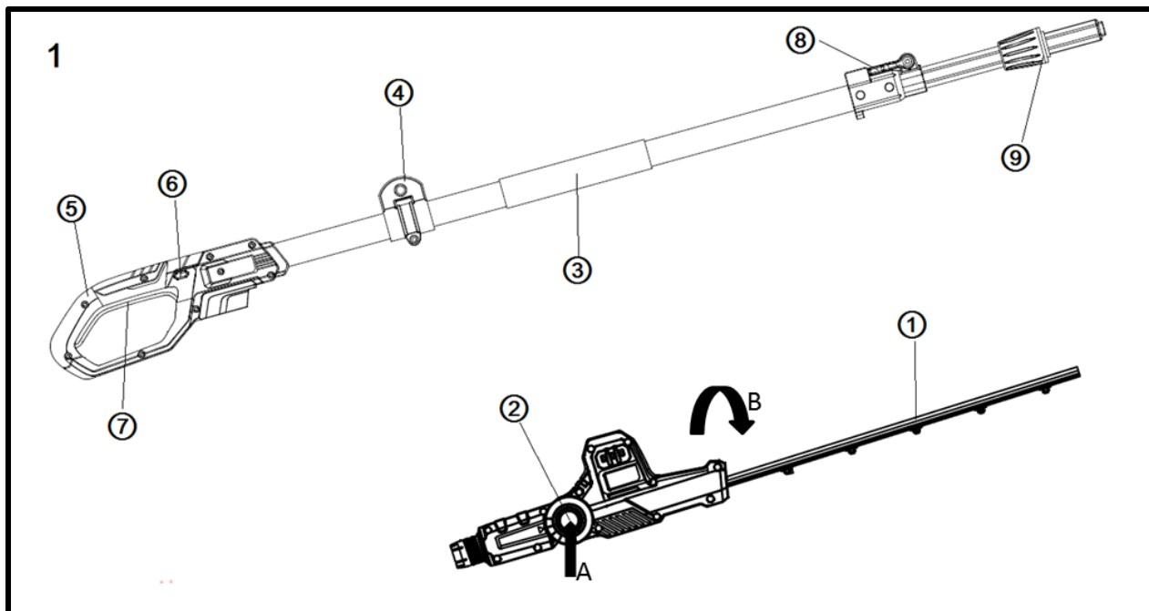
Obrázek 1: Nůžky na vysoké živé ploty
