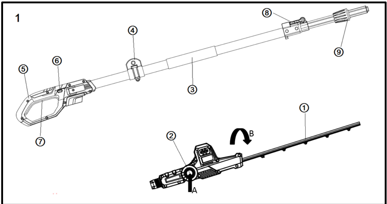
Obrázok 1: Nožnice na vysoké živé ploty
