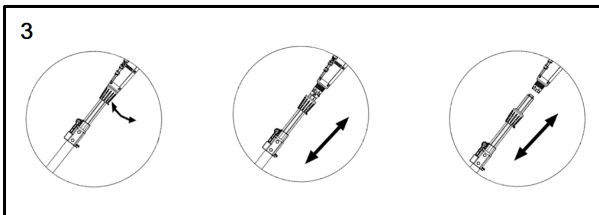
Obrázok 3: Demontáž motora s rezacou hlavou z teleskopického ramena na úsporu miesta pri skladovaní alebo prepravu.
