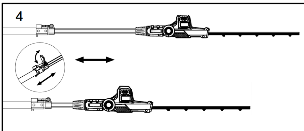
Obrázek 4: Ovládání teleskopického prodloužení
