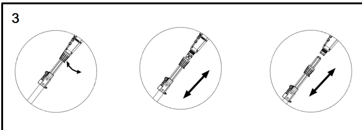
Figura 3: Desinstalação do motor com cabeça de corte da articulação telescópica para armazenamento ou transporte com economia de espaço.
