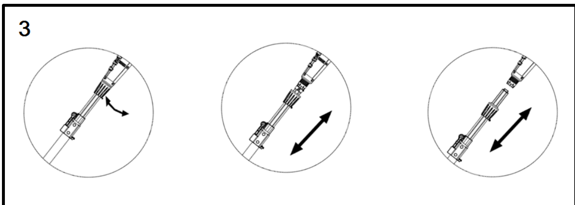
Figuur 3: De motor met snijkop van het telescoopstangenstelsel verwijderen voor ruimtebesparende opslag of transport.
