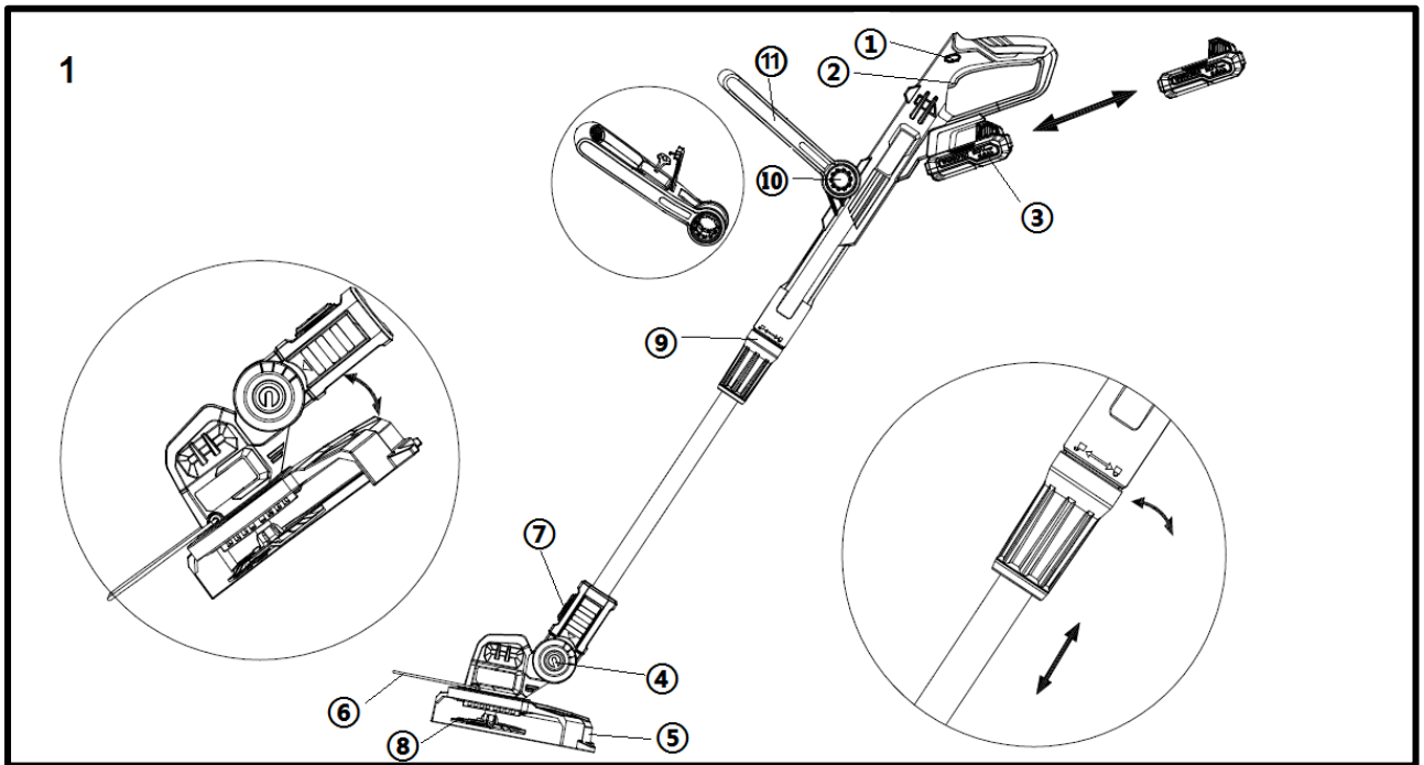
Bild 1: Grästrimmer
