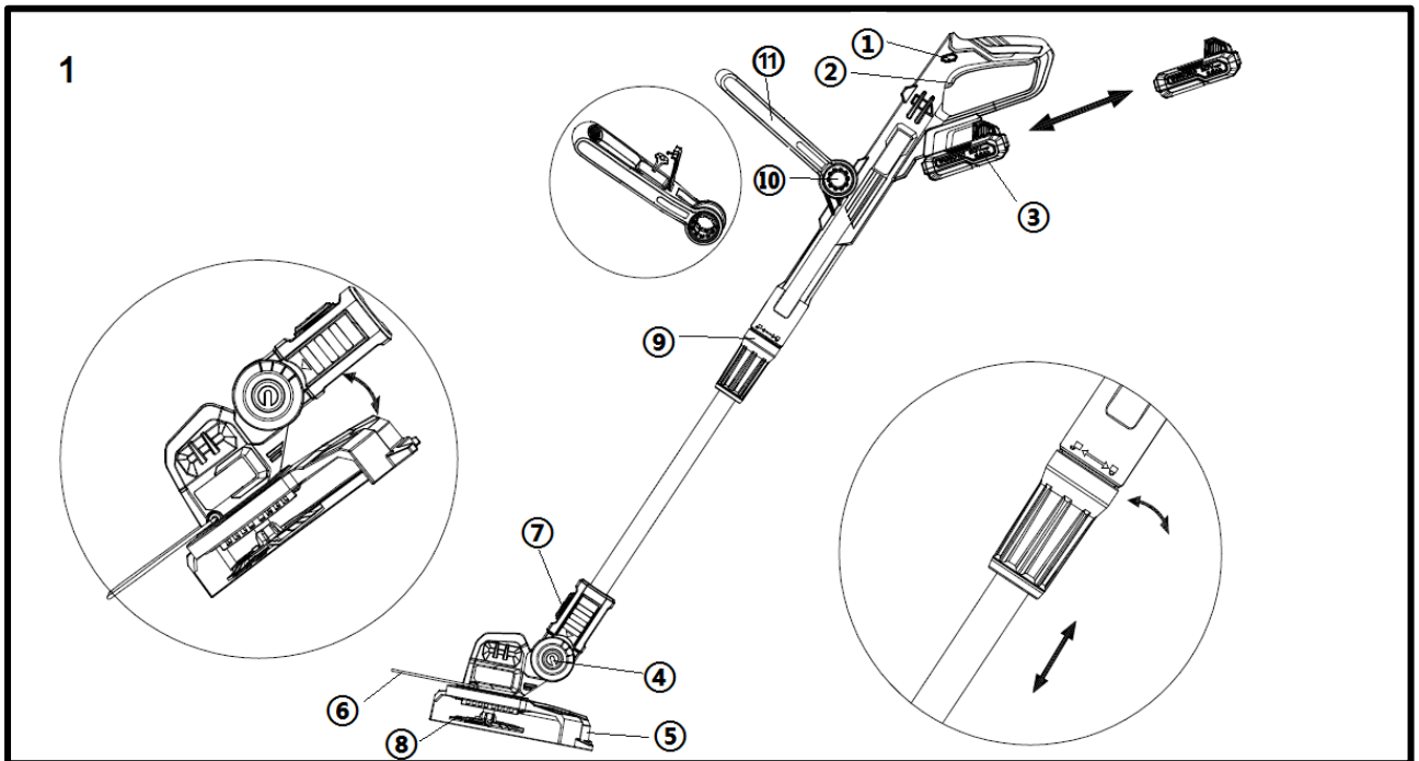
Figure 1 : coupe-bordures
