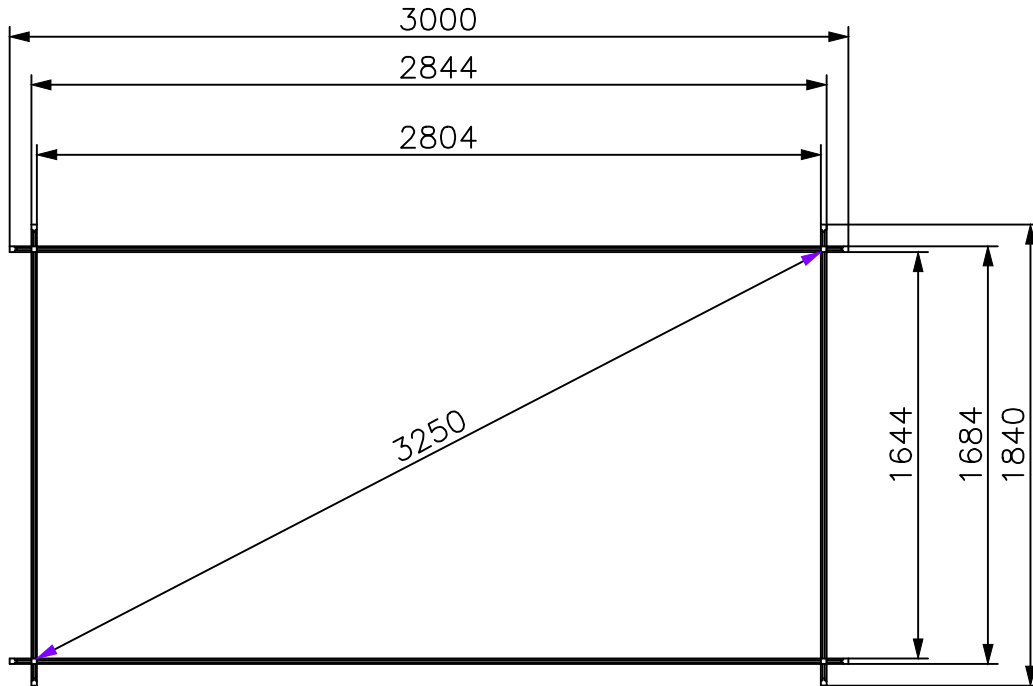
Plan au sol
