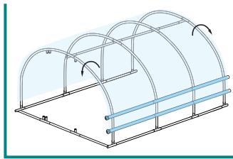
Bâche avec aérations latérales
