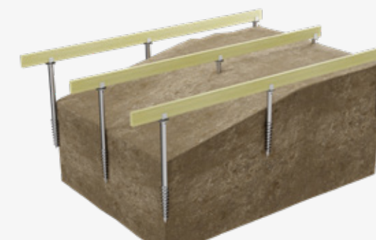
Etape 2 Pose des solives
