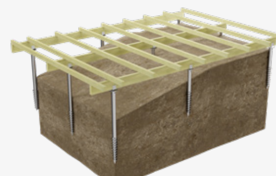
Etape 1 Pose des lambourdes
