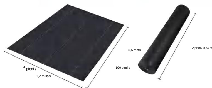
Dimensioni della confezione piegata La larghezza del prodotto è piegata a metà e arrotolata
