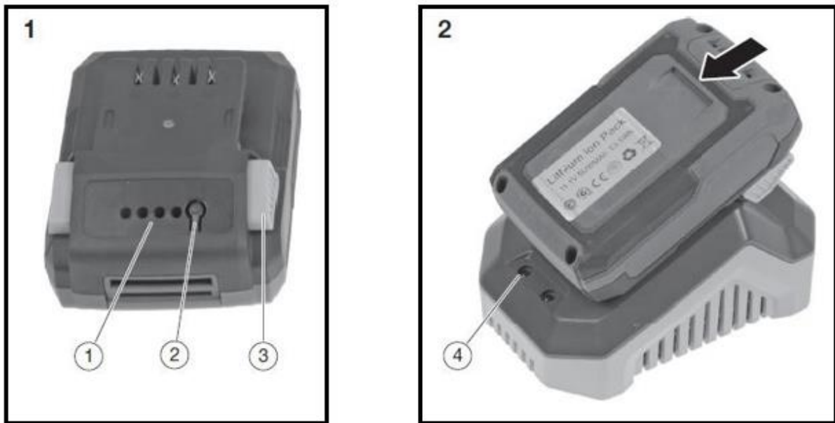
Figura 2: Batteria e Caricabatterie (Caricabatterie come mostrato a destra incluso nella fornitura)
